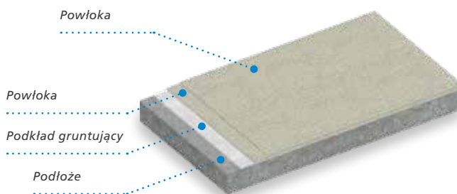
Budowa systemu Triflex CPS-I+
