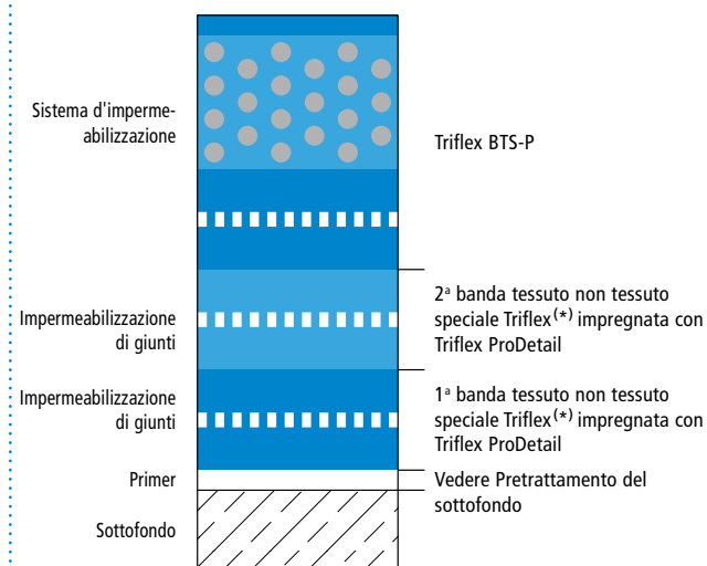
Struttura del sistema – Dettaglio D
