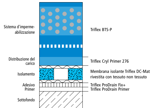
Struttura del sistema – Dettaglio A
