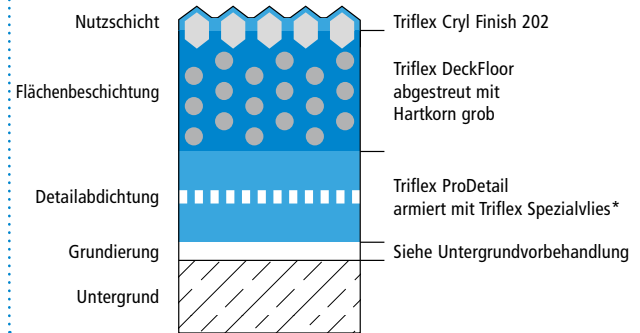
Systemaufbau, Variante 3 – Detail
