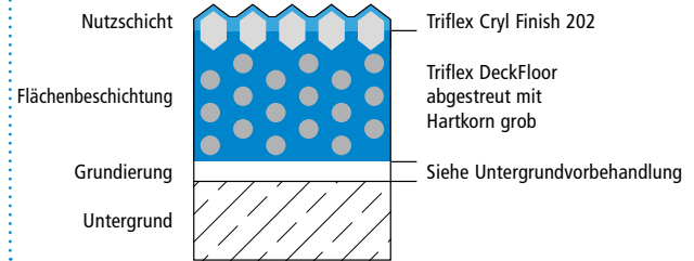
Systemaufbau, Variante 3 – Detail
