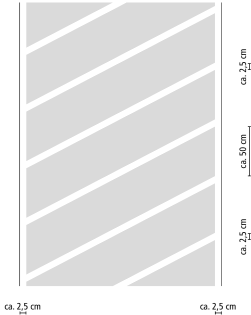
Zeichnung Nr.: DeckFloor-1203
