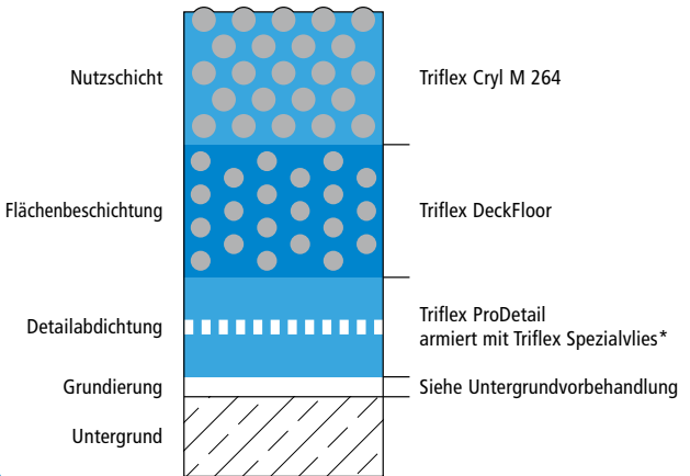
Systemaufbau, Variante 2 – Detail
