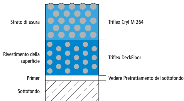
Struttura del sistema – Dettaglio B
