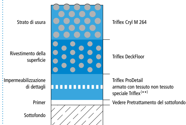
Struttura del sistema – Dettaglio E
