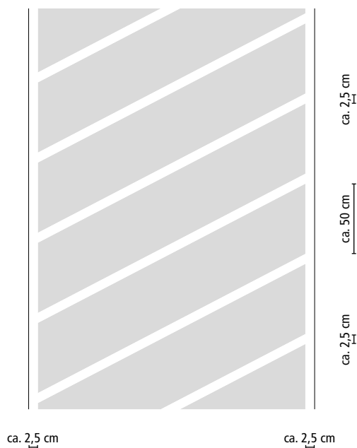
Suddivisione della superficie rampa
