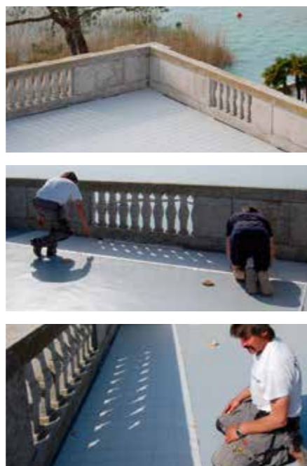
Herzstück des Systems ist eine Folie, die auf den vorbereiteten Untergrund geklebt und ausgeprägt wird. Im Anschluss wird die Folie entfernt und die gestaltete Oberfläche wird sichtbar.
